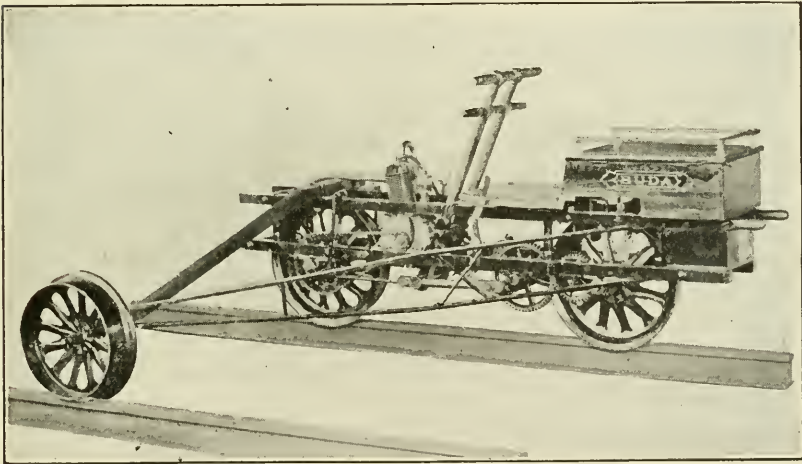
Fig. 1. Light Motor-Velocipede.
